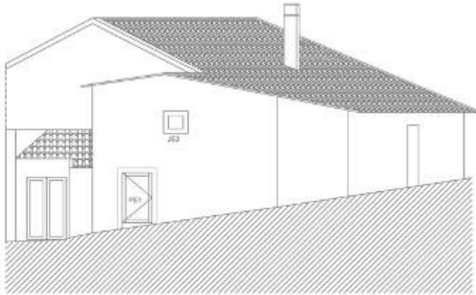
Alçado Lateral
